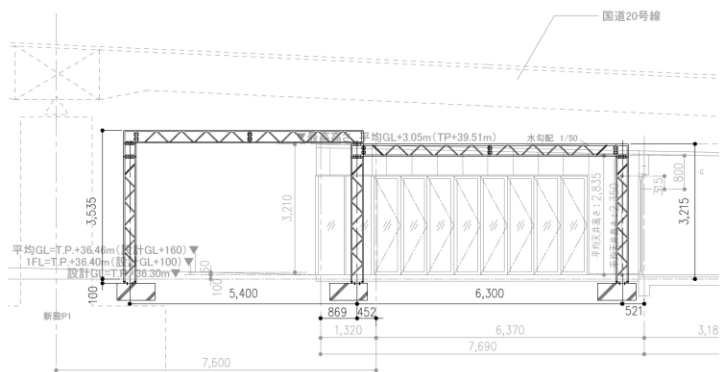
■トラス設置断面図
