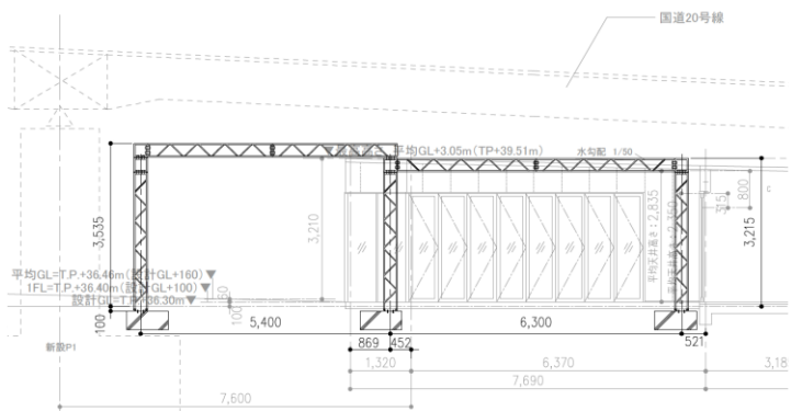
■トラス設置断面図
